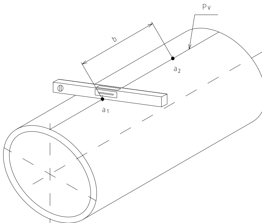
Рисунок 14 Маркировка верхней линии поверхности на измеряемом трубопроводе
