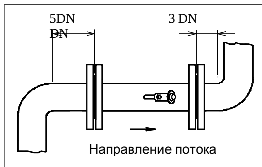
Рис. 7 – Минимальная длина прямых участков трубопровода
