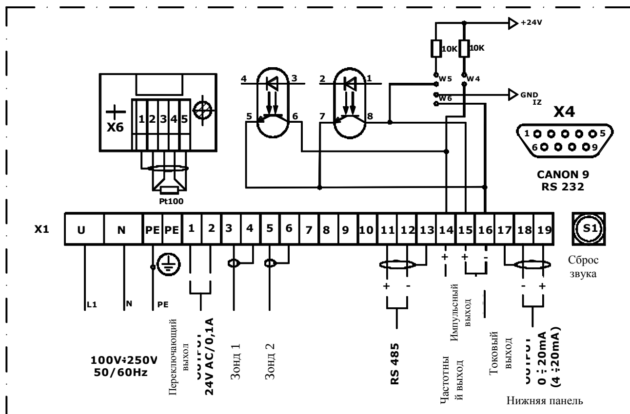
Рис. 15а - Схематическое изображение соединений с ультразвуковым расходомером SE4015
