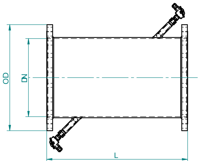
Рис.2 – Размерная схема датчика расходомера
