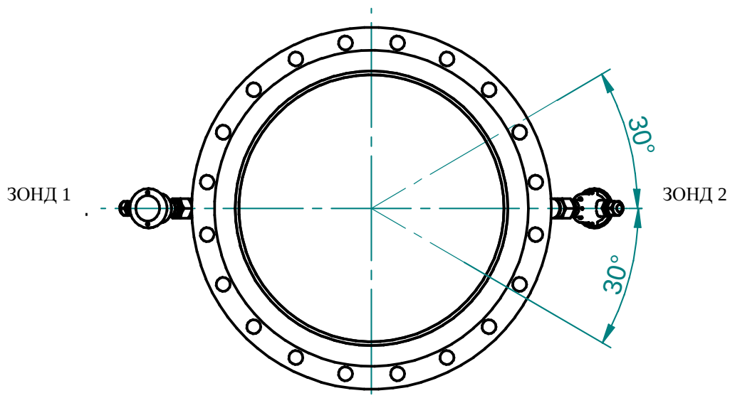
Рис. 13а - Допустимый диапазон поворота однолучевого датчика по отношению к его продольной оси (SE4015)
