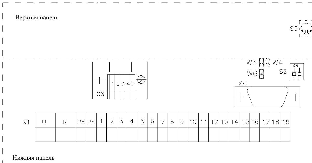
Рис. 16 – Расположение переключателей S2 и S3
