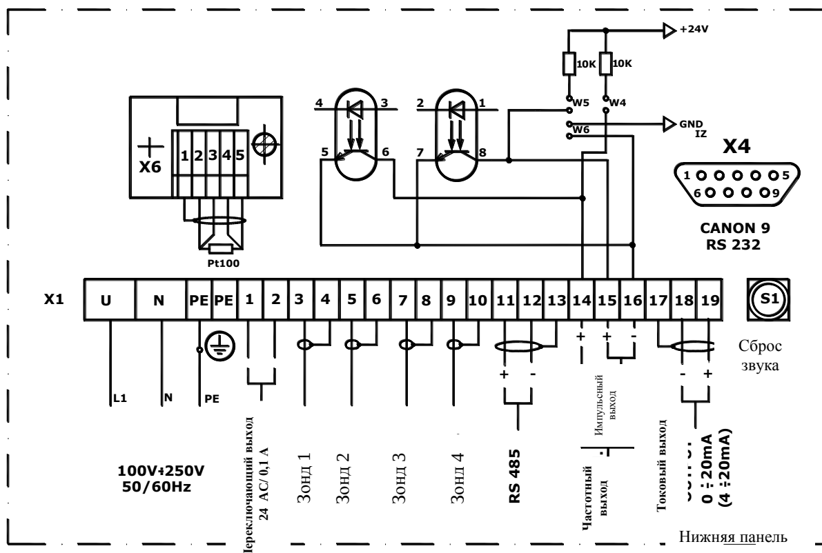
Рис. 15б - Схематическое изображение соединений с ультразвуковым расходомером SE4025
