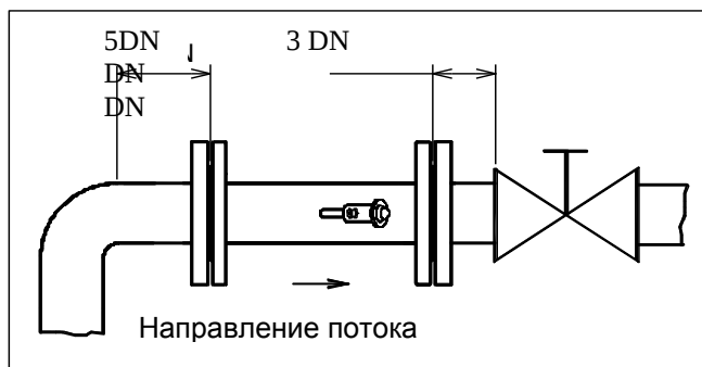
Рис. 8 – Минимальная длина прямых участков трубопровода на участках со стороны задвижки
