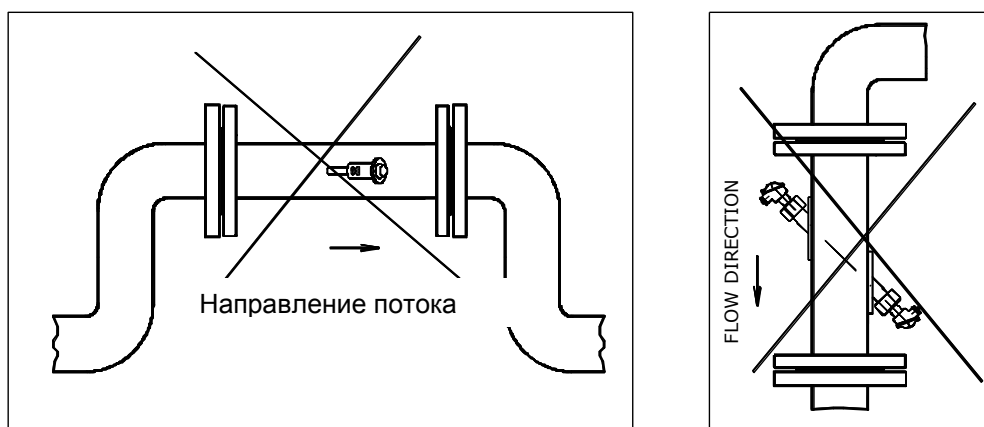
Рис. 12 – Примеры неправильного размещения датчика
