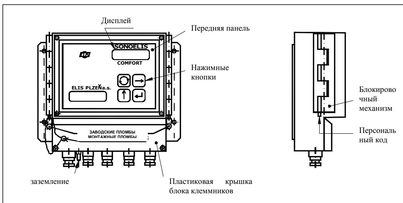
Рис. 5 – Электронный блок - описание
