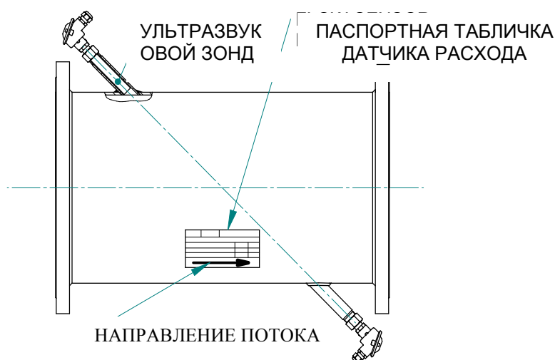
Рис. 4 – Ультразвуковой датчик - описание
