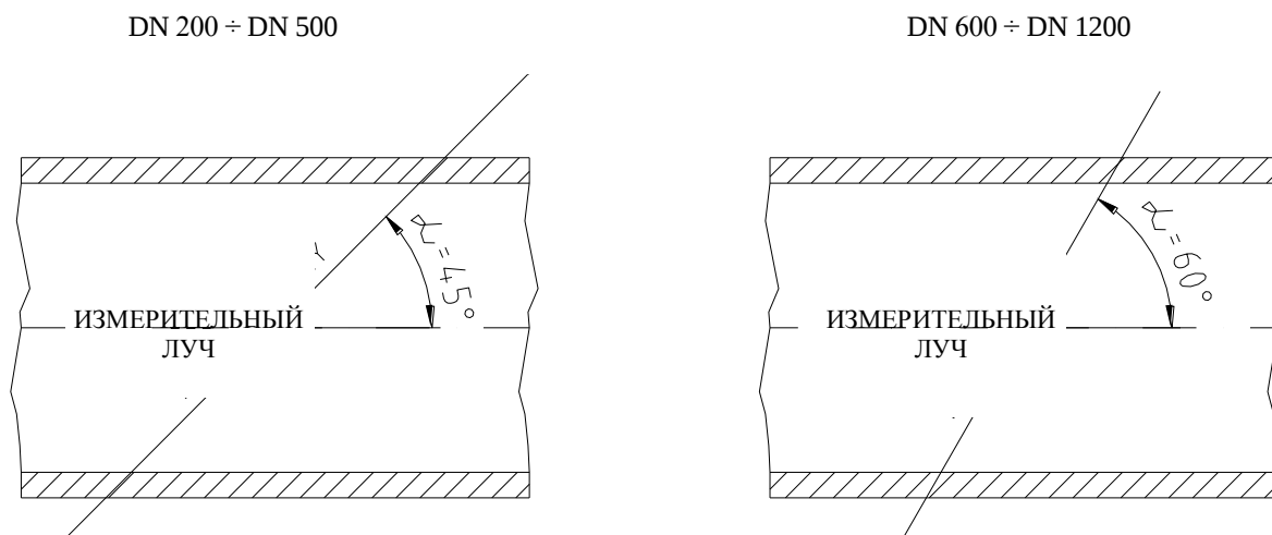
Рис.1 – Ультразвуковой угол ориентации луча относительно оси трубопровода
