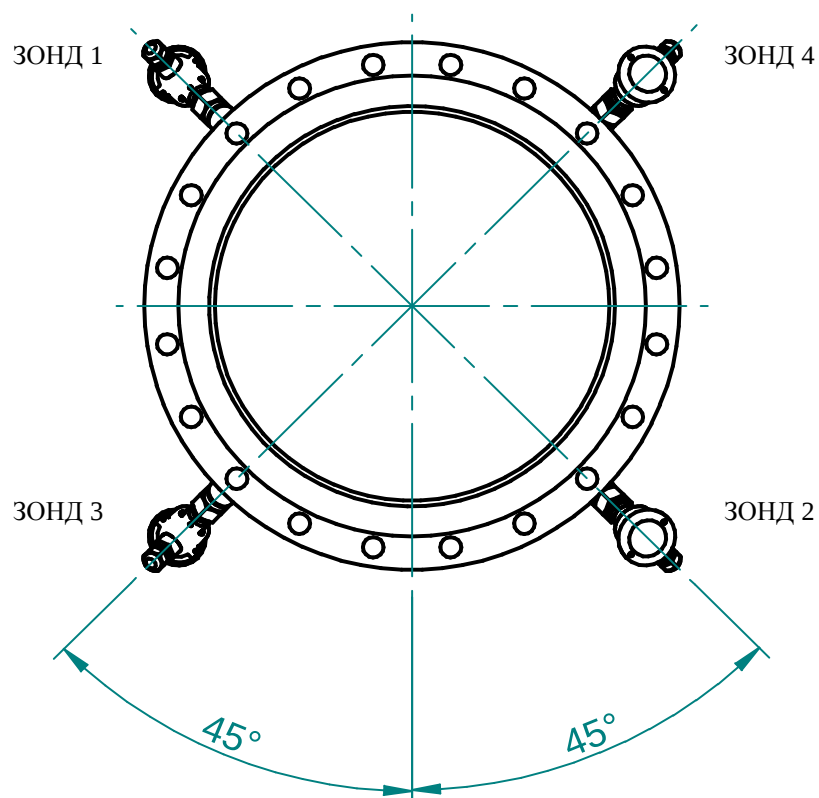
Рис. 13б - Угол между плоскостями зондов и вертикальной плоскостью с двухлучевым датчиком (SE4025)
