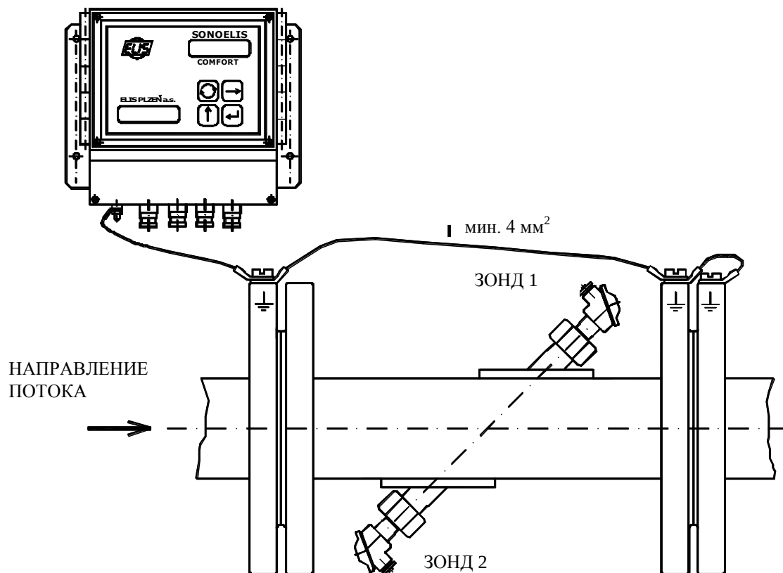
Рис. 14 – Заземление электронного блока и датчика расходомера
