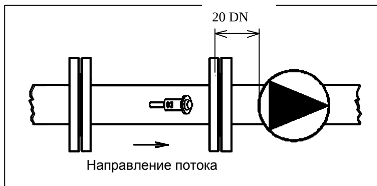
Рис. 9 - Минимальная длина прямого участка трубопровода до насоса
