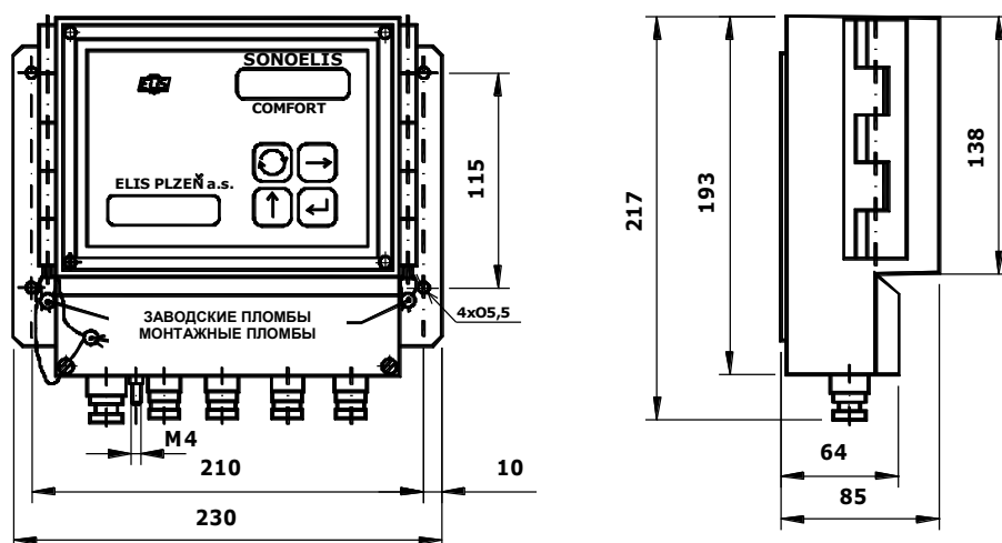
Рис. 3 – Габаритные размеры электронного блока
