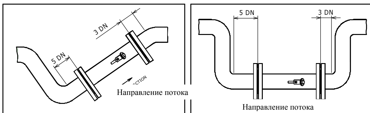
Рис. 10 – Расположение датчика, обеспечивающее полное затопление в любое время
