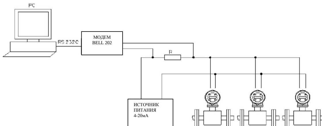
На рисунке ниже показана типичная многоточечная сеть.
