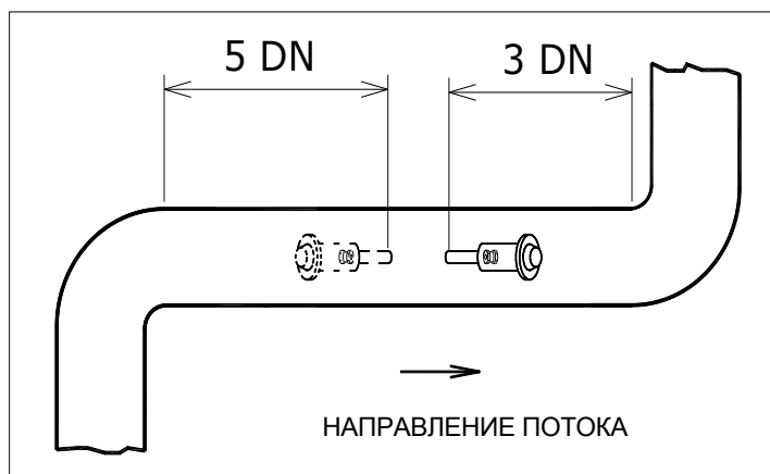
Рис. 13 Рекомендуемые размеры секции трубопровода со стабильным течением жидкости перед и после ультразвукового расходомера
