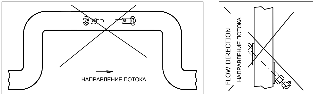
Рис. 18 Примеры неправильного размещения датчика
