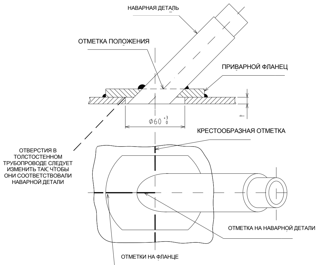
Рис. 23 Сборка наварных деталей
