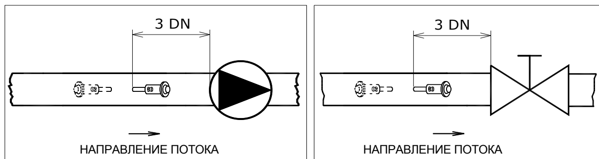
Рис. 15 Прямые участки трубопровода для устранения воздействия возмущений на стороне выхода датчика
