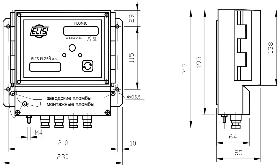
Размерная схема короба электронного блока
