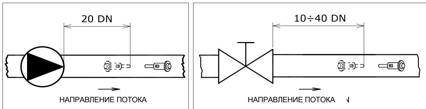
Рис. 14 Прямые участки трубопровода для устранения воздействия возмущений на стороне входа датчика
