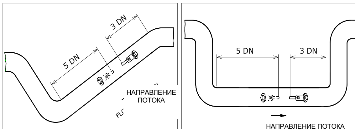
Рис. 16 Размещение датчика в нижних коленах, гарантирующих полное заполнение все время проведения измерений
