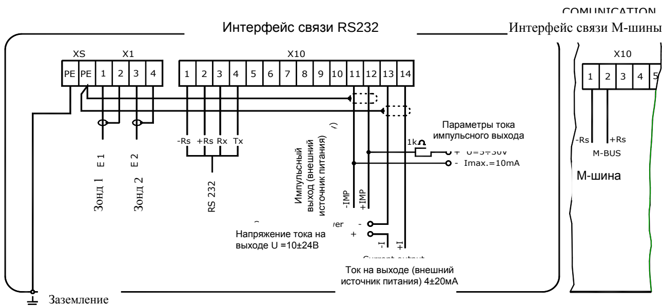
Рис. 29 Входные и выходные сигнальные соединения электронного блока UP 8.00
