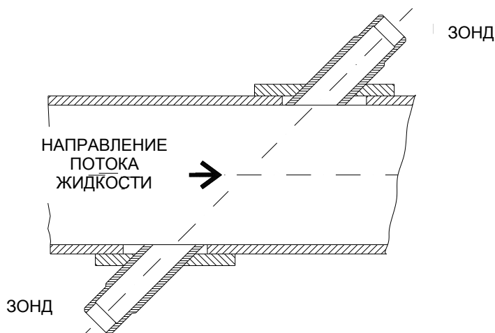
Рис. 30 Маркировка зондов
